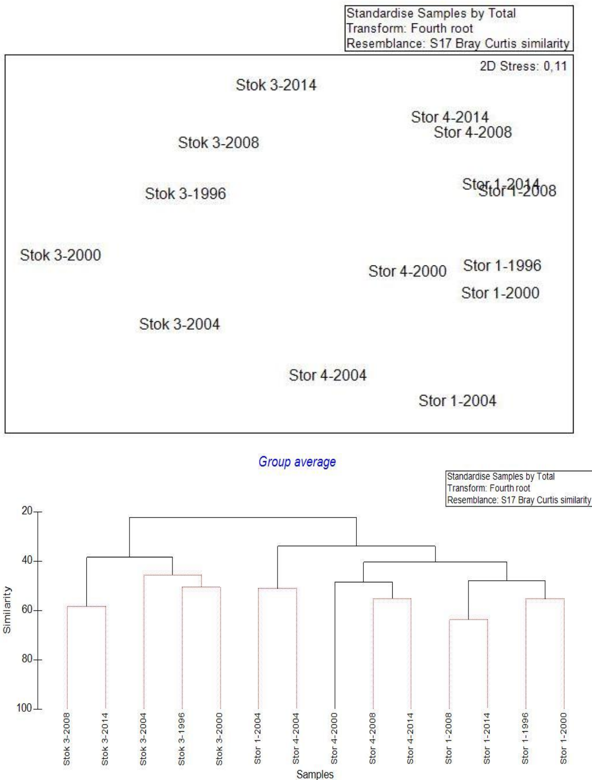
Figur 3.7: Cluster plot på hugg-nivå fra Svartasmoget. Beregningene er foretatt på standardiserte og fjerderots-transformerte artsdata. Basert på Bray-Curtis indeks. Plot viser faunalikhet mellom de undersøkte stasjonene.
