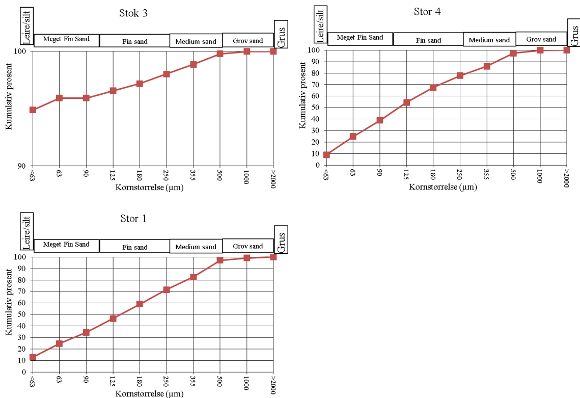
Figur 3.5. Kornfordelingskurver fra sedimentet på de undersøkte stasjonene i 2014. Y-aksen viser prosentvis fordeling av de forskjellige kornstørrelsene.
